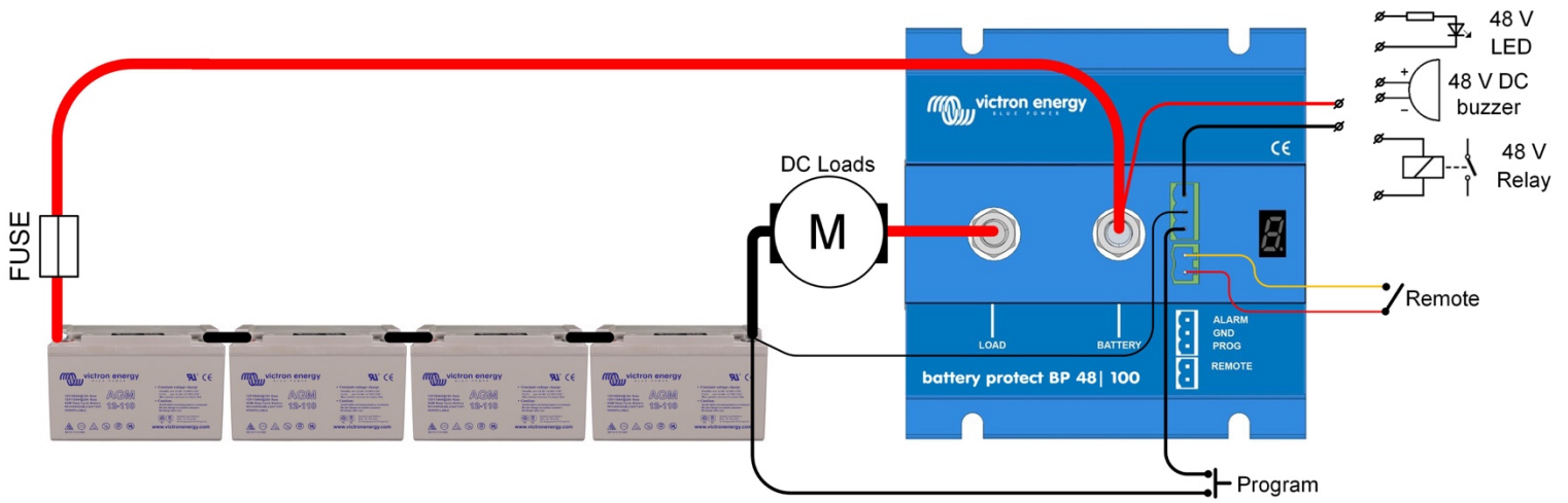
Kopplingschema för BP 48|100
